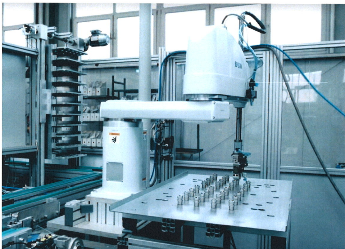
Foto: Automatizace vstřikovacích lisů pro výrobu tvarovek s kovovými zástřiky
